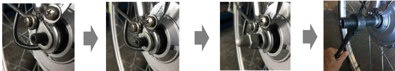
④前ホーク爪部 左右ともに 前輪脱落防止金具、ワッシャー、袋ナットの順に組付け 前車輪と前ホークの間隔 車輪タイヤ位置を確認しながら ナットを30~40N/mのトルクで締め付けてください
