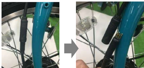
②カバーを外すとコードジョイントコネクターが現れる、ジョイントコネクターを引き抜きます。
