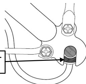
③前ホーク爪溝に爪付きカラーの凸部を合わせて前ホーク爪溝に沿って差し込みます、軸から出ているモーターコードが下側から出るようになります。
